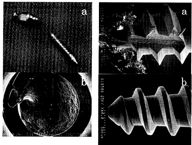
図1. (a) 撤去時に破断した矯正用ミニスクリューインプラント, (b) そのSEM像
